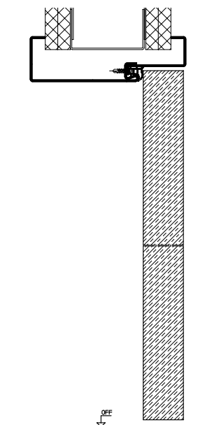
Huisserie enveloppante à hauteur d'étage préparée en option pour faux-linteau
