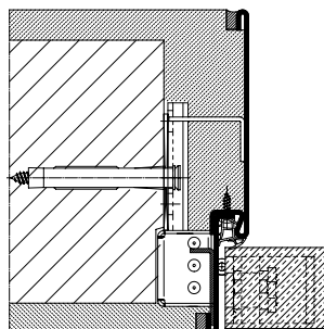
Huisserie en 2 parties sans recouvrement, affleurante, pour maçonnerie, avec paumelle masquée
