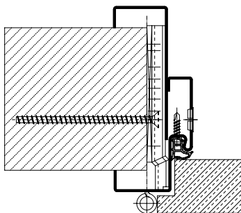
Huisserie télescopique en 2 parties sans ajustement de l'huisserie, avec recouvrement de feuillure .NOUVEAU
