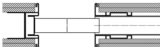
Huisserie de porte coulissante sans recouvrement à galandage
