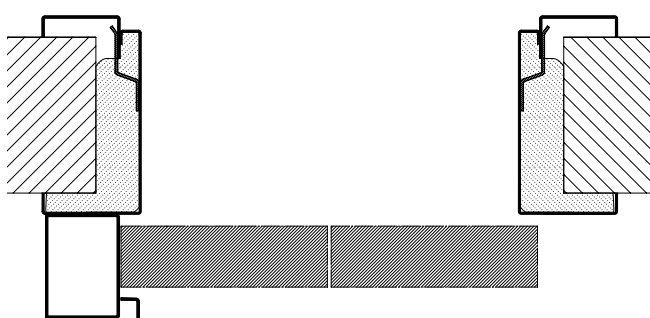
Huisserie de porte coulissante VarioFix en applique
