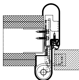
Huisserie en 2 parties « Roundstyle », affleurante, pour ossature métallique avec sécurité antipincement côté paumelles
