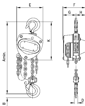
Modell VS///, 250 - 3.000 kg, einsträngig
