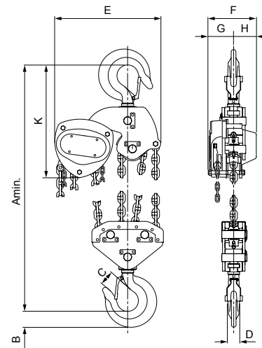
Modell VS///, 10.000 kg, viersträngig
