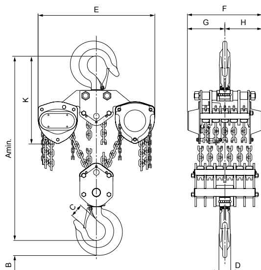
Modell VS///, 30.000 kg, zwölfsträngig
