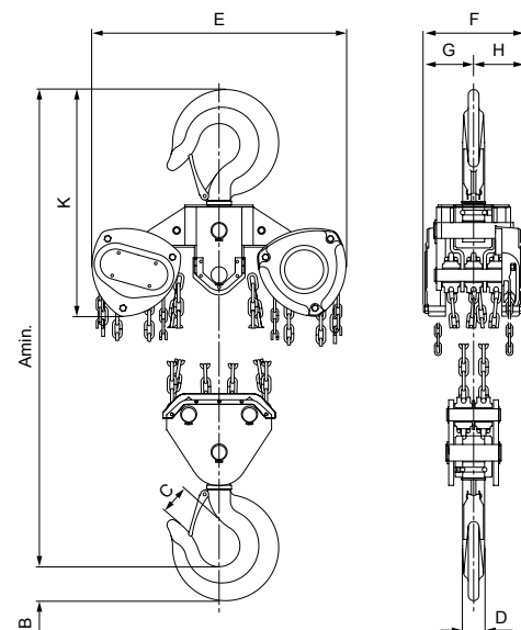
Modell VS///, 20.000 kg, achtsträngig
