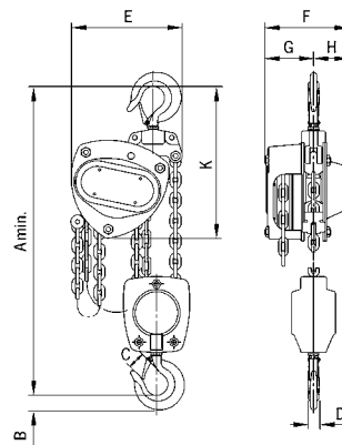
Modell VS///, 2.000 - 5.000 kg, zweisträngig
