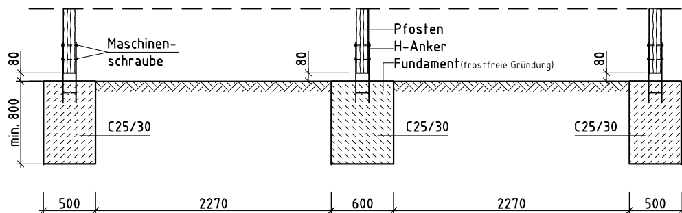
Schnitt A-A M1:50
