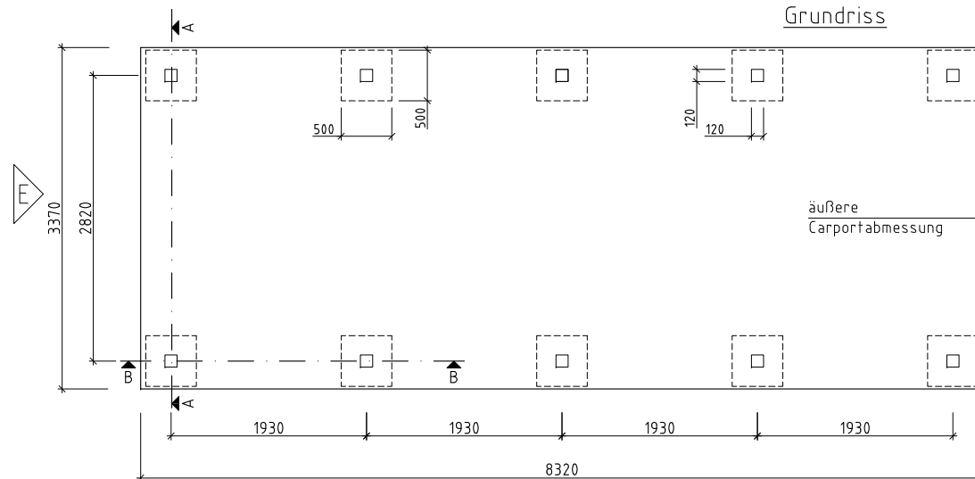
Grundriss
