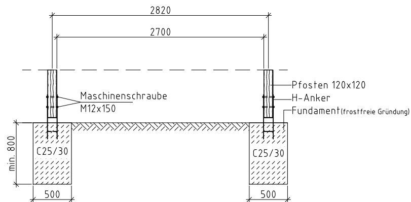
Schnitt A-A
