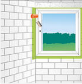
Bild 10: Folie mit Andruckroller anrollen
