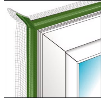
Bild 5: Folie im Eckbereich falten
