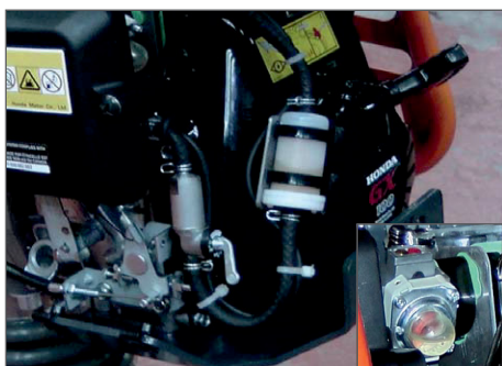
2-faches Treibstofffilter System & Vergaser mit Primer Pumpe für einen schnellen Startvorgang.
