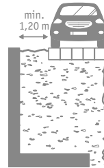
E | Verkehrslast bis p = 5 \text{ kN/m}^2 , mit Ver- dichtungserddruck e_{vh} = 25 \text{ kN/m}^2 , Abstand: 1,2 m (bis 155 cm Höhe)/ 1,5 m (ab 180 cm Höhe) (55-105 cm Höhe ausgenommen)
