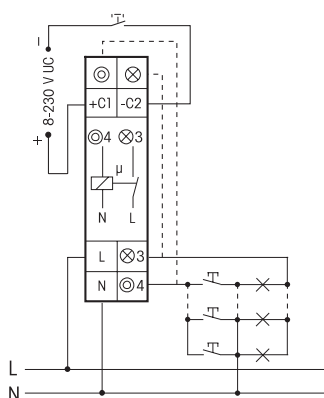
3-Leiter-Schaltung, nachschaltbar.
