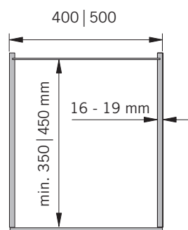
Aufsicht/Top view
