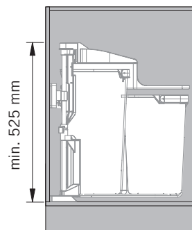
Vorderansicht/Front view
