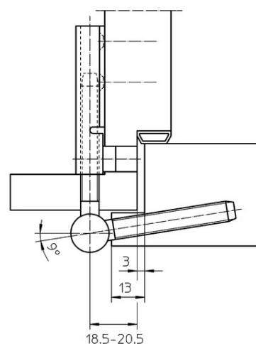
Querschnitt
