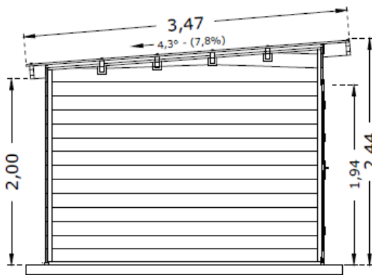
Schnitt / section
