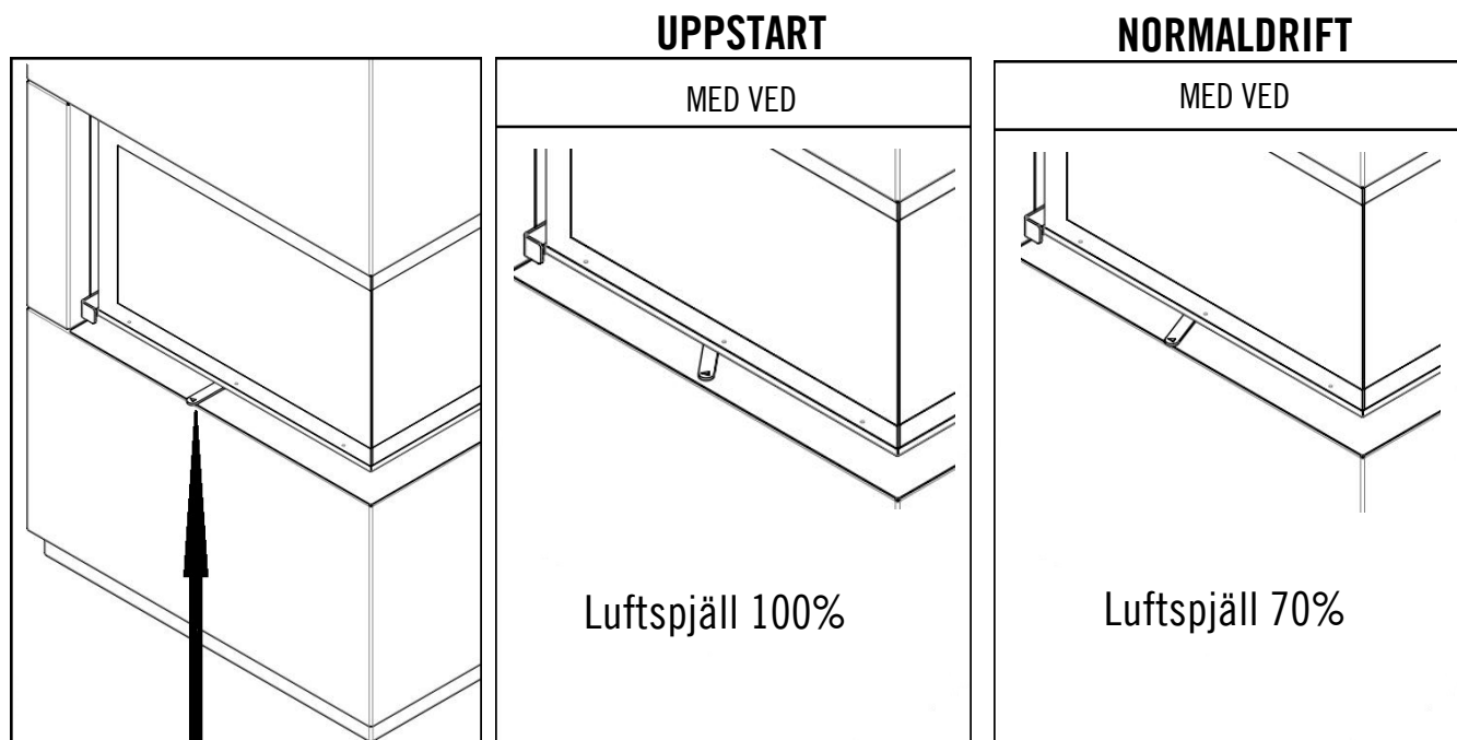
Figur 7 – Användning av luftregleraren
