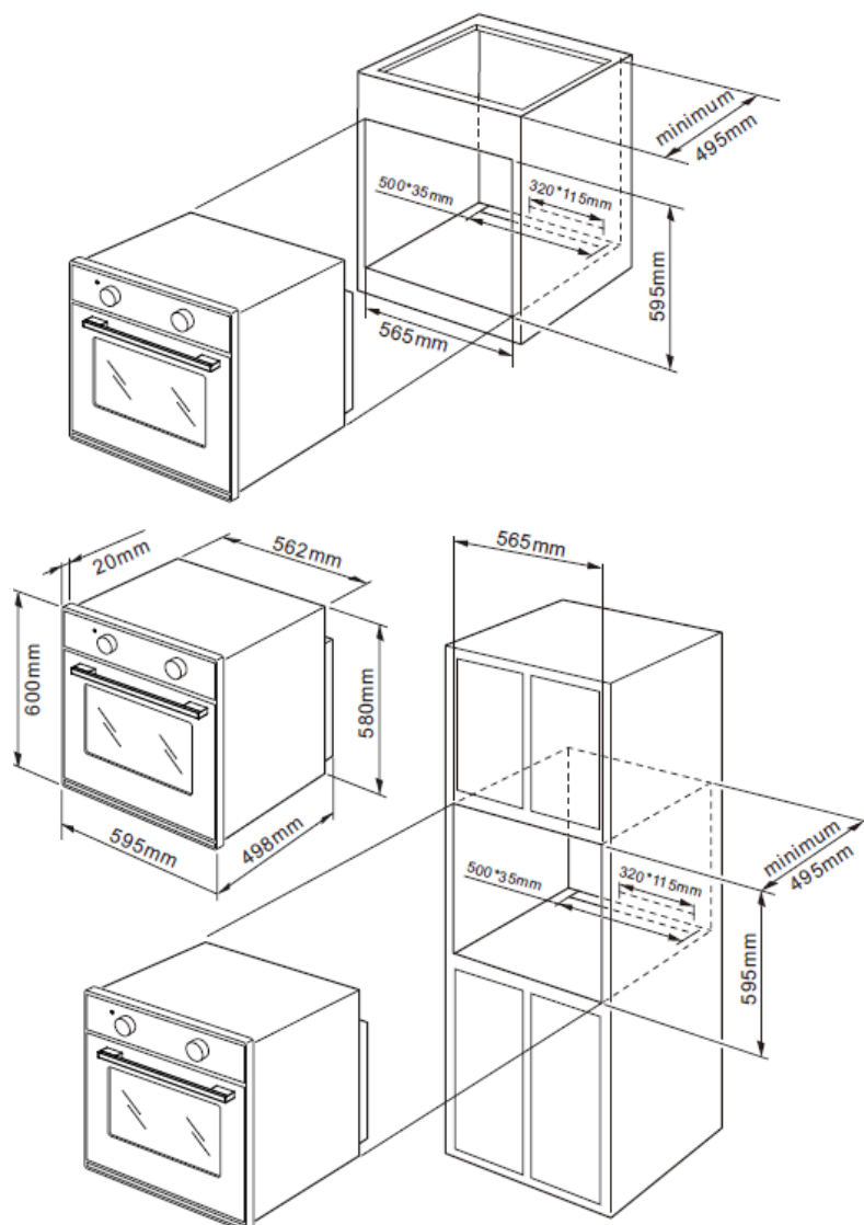
ABB. 1: INSTALLATIONSZEICHNUNG
