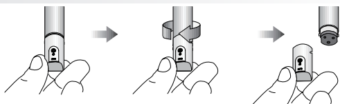
Demontáž trysky (proti směru hodinových ručiček)
