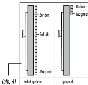
Positionering rolluik-zender (zij aanzicht)
