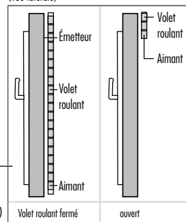
Positionnement de l'émetteur pour volet roulant (vue latérale)
