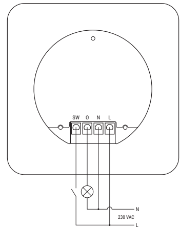
Wiring diagram / Schaltplan / Diagramma di cablaggio
