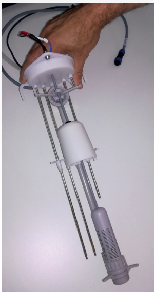
Elektrodenatz
