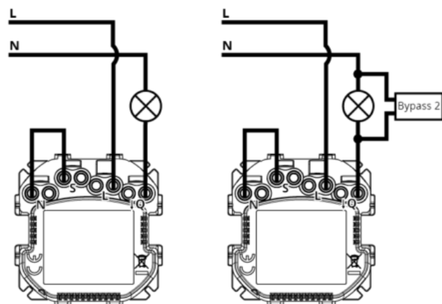
Diagramm 2: Anschlussbeispiel für 3-Leiter-Installation mit Bypass 2
