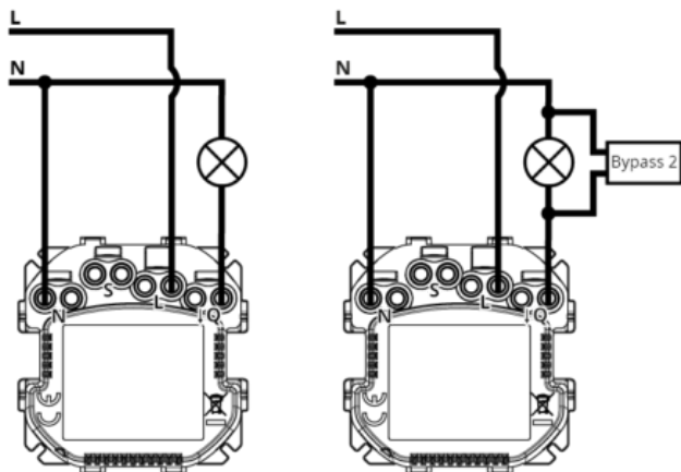
Diagramm 1: Anschlussbeispiel für 3-Leiter-Installation
