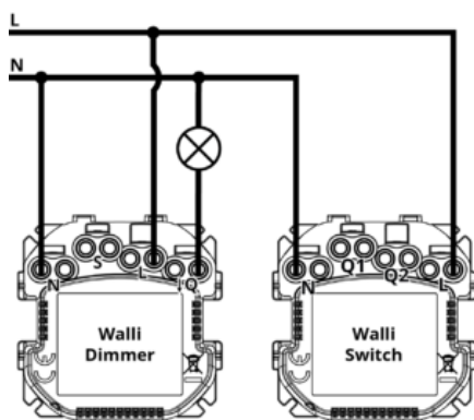
1. 3-Leiter Installation
