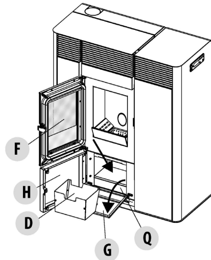
Fig. 17 - Entnahme Brennschale
