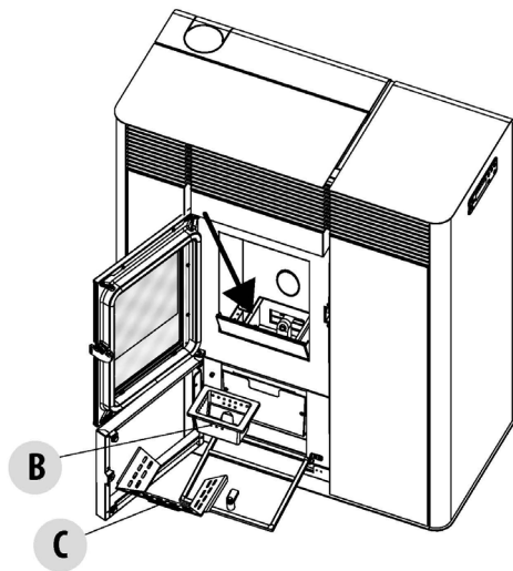
Fig. 16 - Entnahme Aschenlade
