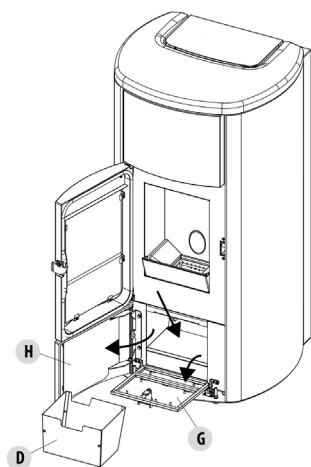
Fig. 14 - Entnahme Aschenlade
