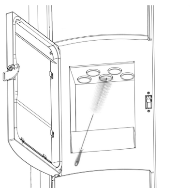
Fig. 20 - Reinigung der Rohrbündel
