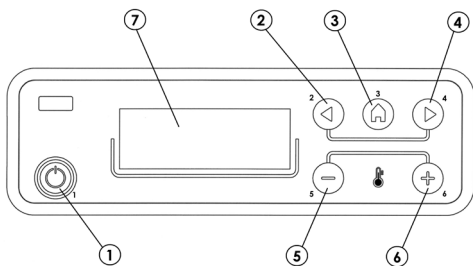
Fig. 2 - Display
