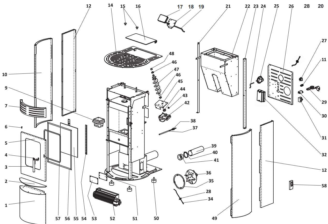
Abb. 14 Explosionszeichnung
