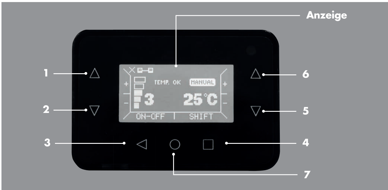
Abb. 3: Steuerungskonsole
