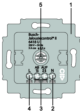
Abb. 2: Geräteansicht
