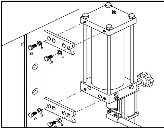
Abb. 12: Pumpeneinheit montieren
