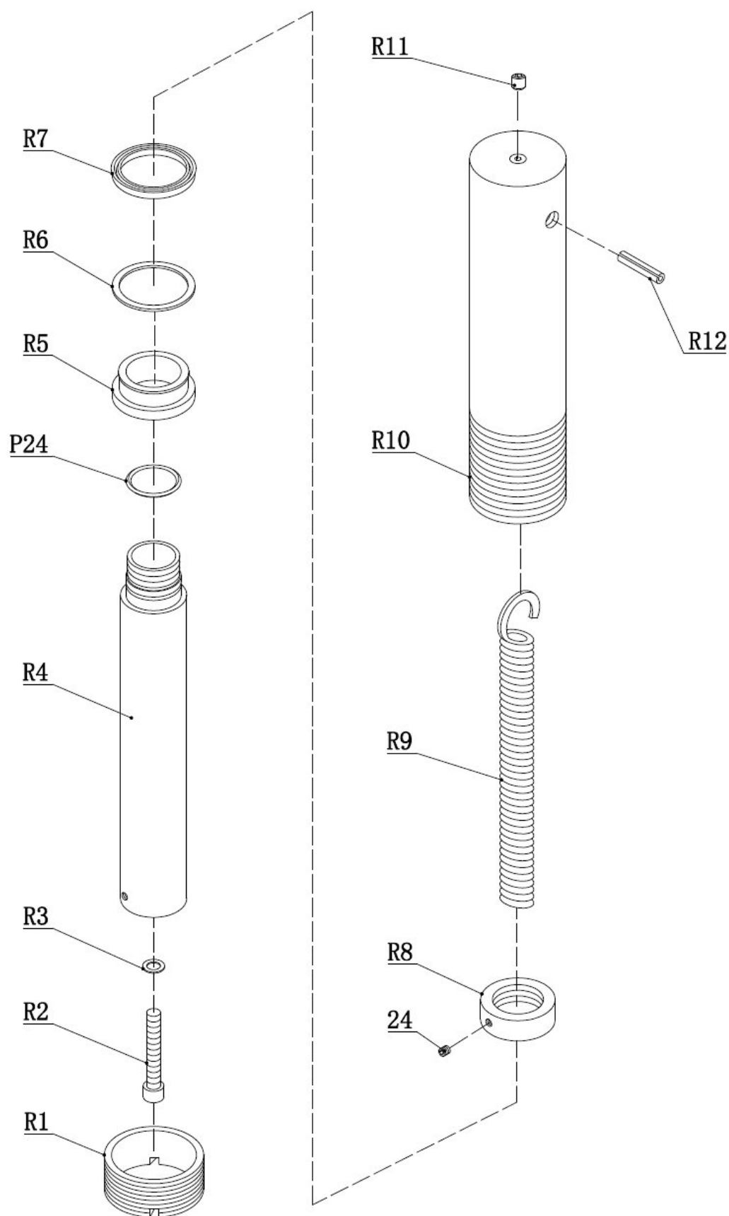
Abb. 18: Ersatzteilzeichnung 2 AWPP 20 E
