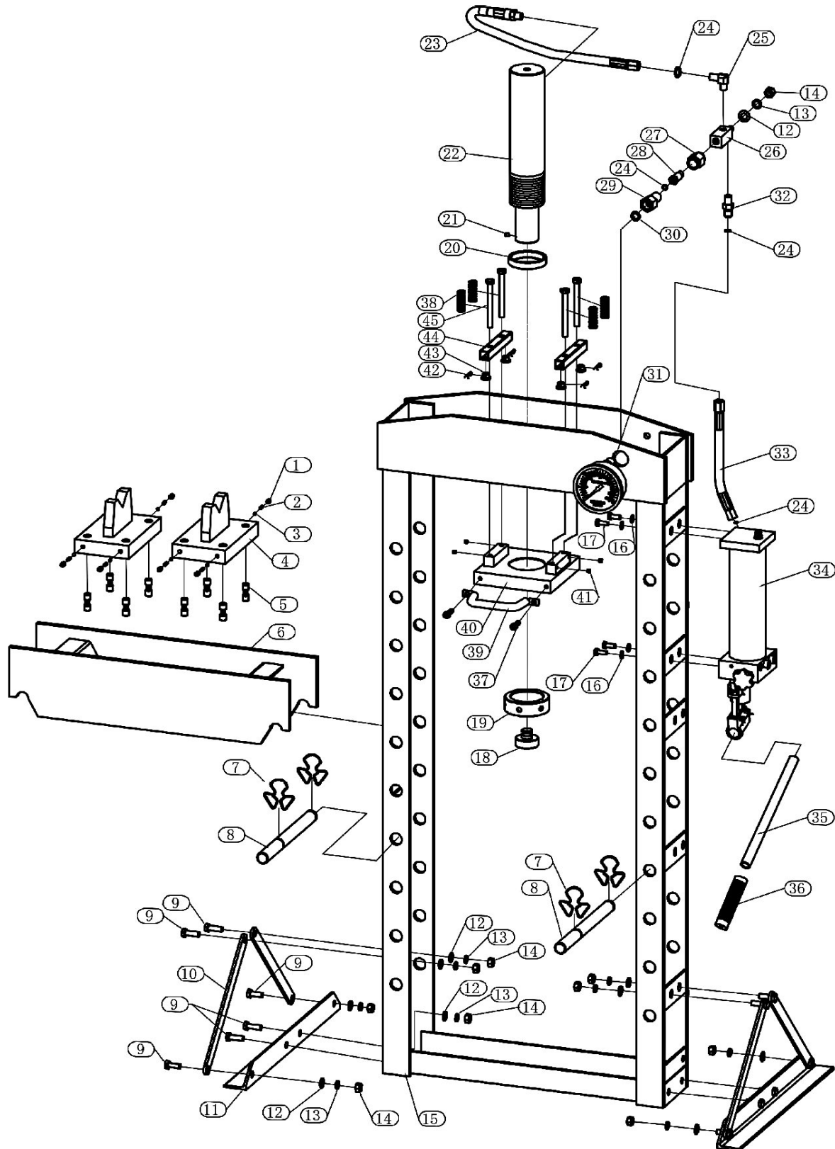
Abb. 17: Ersatzteilzeichnung 1 AWPP 20 E
