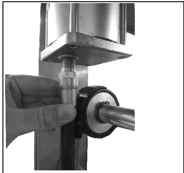
Abb. 15: Druckluftverbindung montieren
