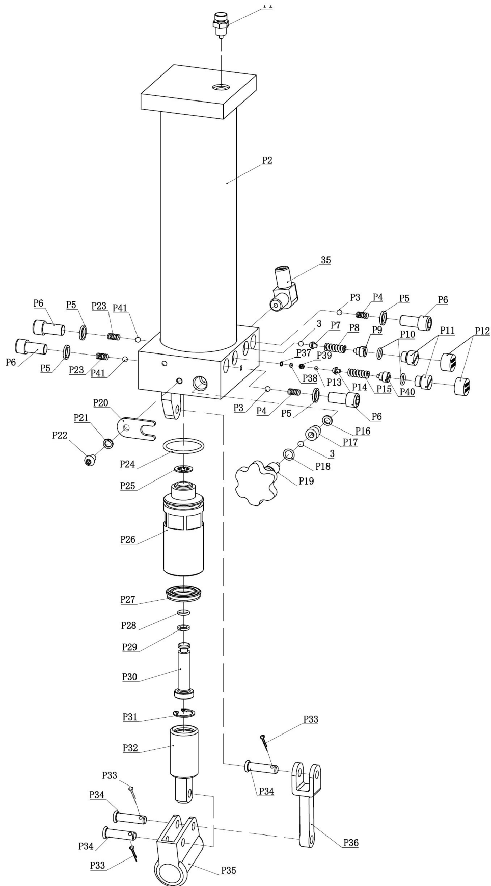
Abb. 19: Ersatzteilzeichnung 3 AWPP 20 E
