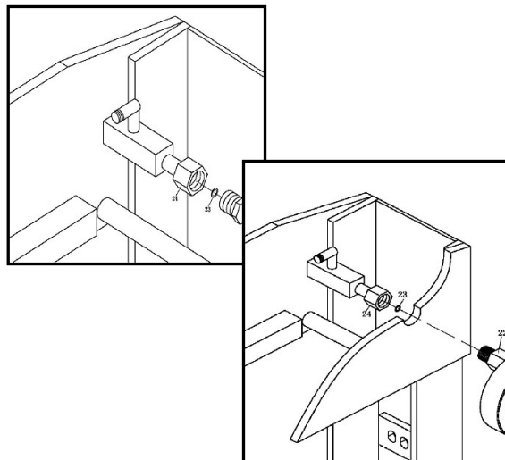
Abb. 9: Manometer montieren
