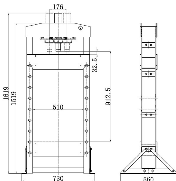
Abb. 2: Abmessungen AWPP 20 E
