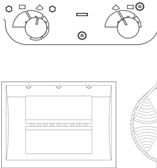
Abbildung 13 – LuftEinstellung und Brennstoffanordnung beim Betrieb mit Scheitholz - Zeitbrandbetrieb
