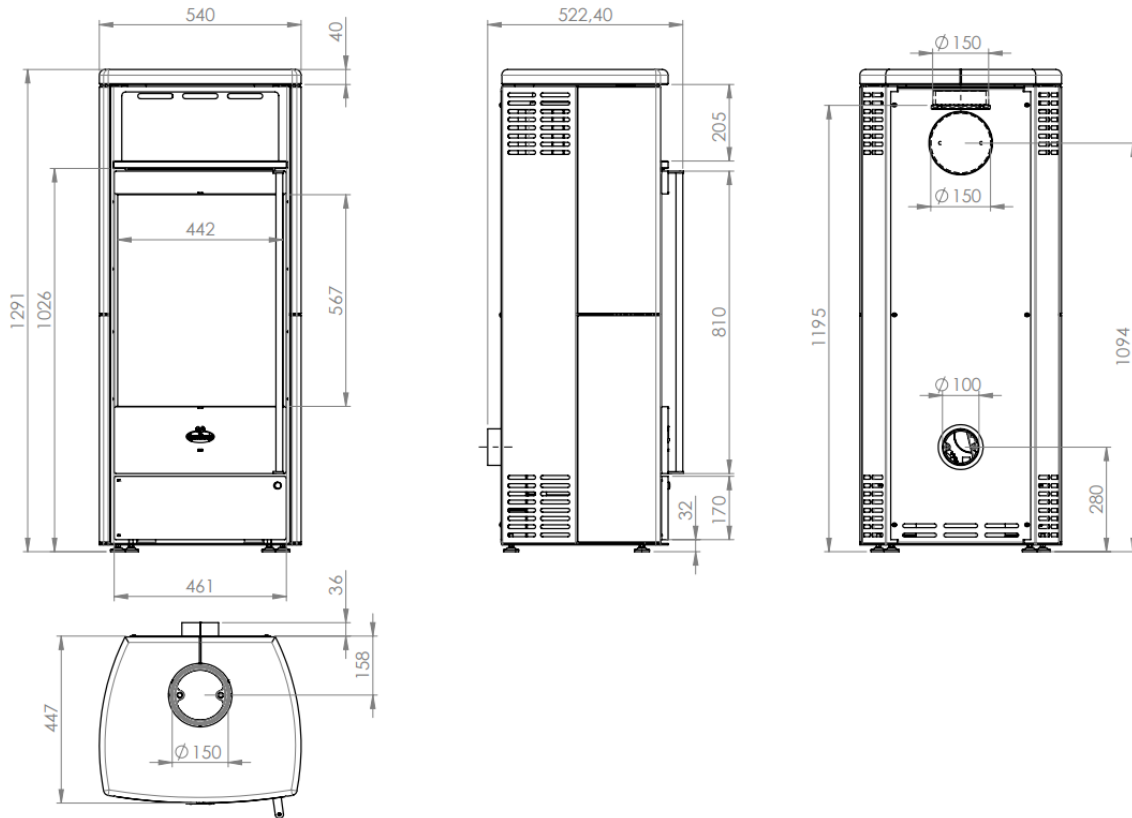
Abbildung 3 – Hauptmaße
