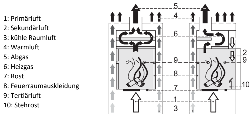
Abbildung 4 – Fire-Plus System, schematische Darstellung
