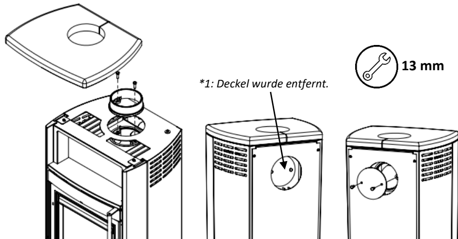
Abbildung 5 - Abgasstutzen und Abdeckung demontieren
