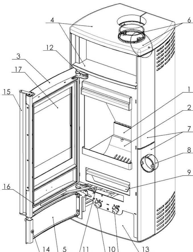
Abbildung 1 – Aufbau des Geräts
