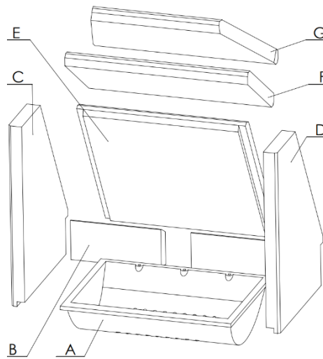
Abbildung 16 – Feuerraumauskleidung mit Rost
