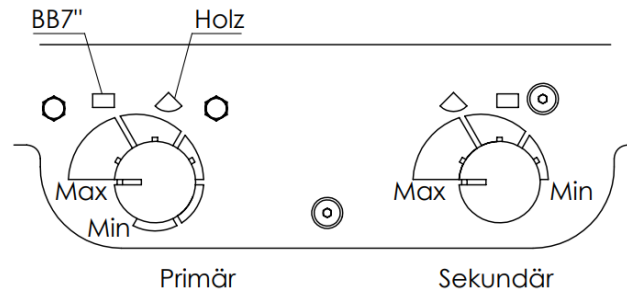
Abbildung 12 - Links: Primärluftregler, rechts: Sekundärluftregler
