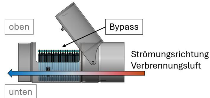
Abbildung 3: Waagerechter Einbau des Culimeta Feinstaubfilter.
