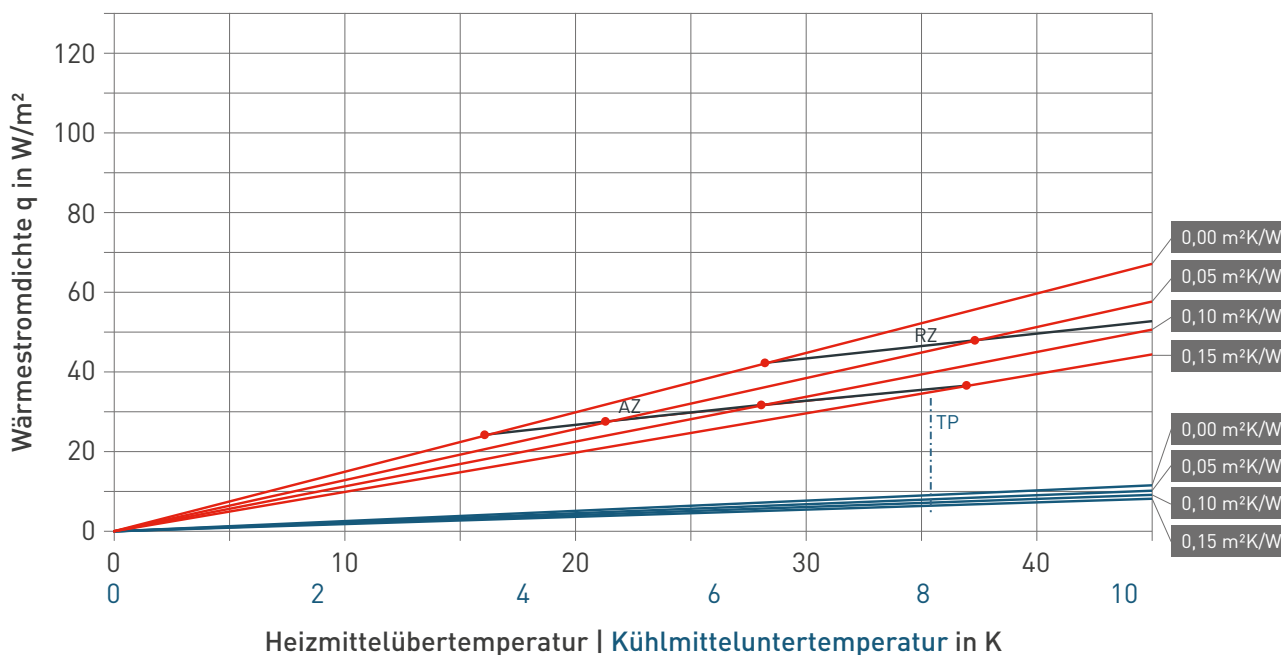
Kennliniendiagramm Heizen und Kühlen fermacell® Therm 25-10, MKV 16x2, VA = 334 mm
