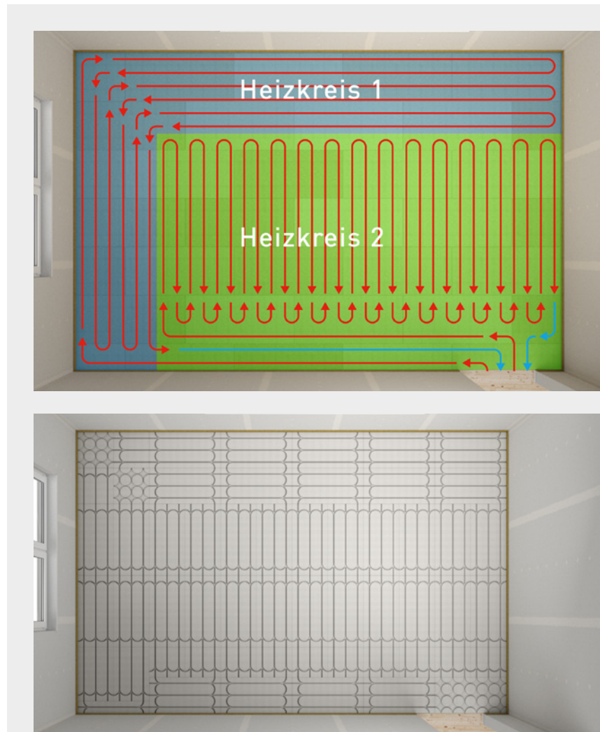
Verlegschema mit zwei Heizkreisen
