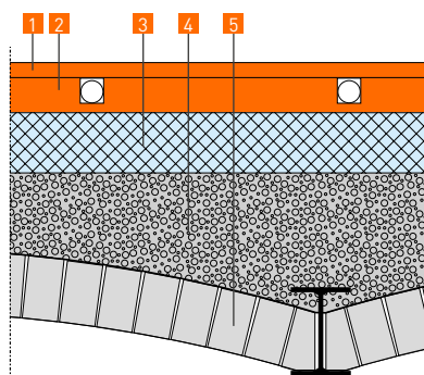
Niveausgleich auf Gewölbedecke mit fermacell® Therm25 (Bauphysik ist zu beachten)
