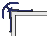
Ecke außen / Eckverbinder auf der Ecke
