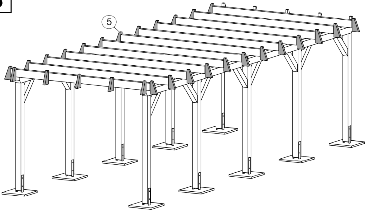
Abbildung Art.-Nr.: 615.3483...
