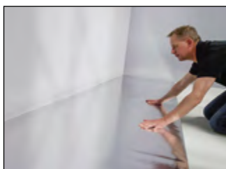
Verlegeunterlage auf vorbereitetem Untergrund auslegen.
