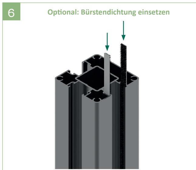
6 | Jeweils zwei Bürstendichtungen in die Pfostennuten einschieben.
