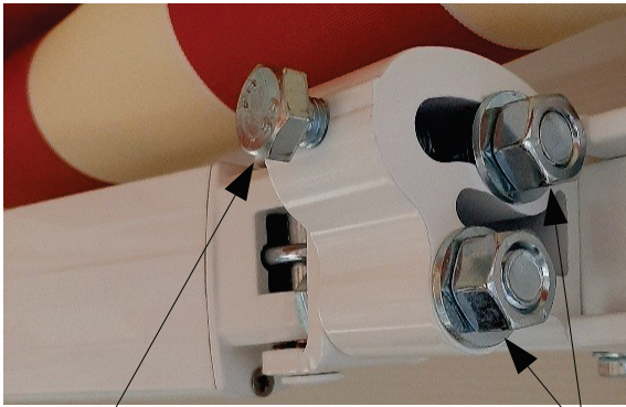
Stützschraube (2)
