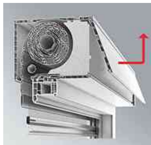
Typ A Expert XT – Revision* innen hinten Kasten innen eckig Putzträger außen möglich
