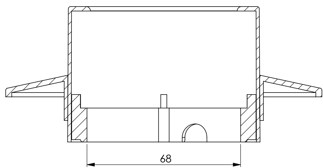
SCHNITT A-A MAßSTAB 1 : 1
