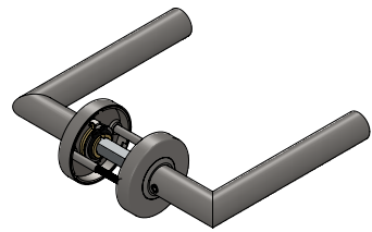
Isometrisch aanzicht Schaal 1:5 0035.058302
