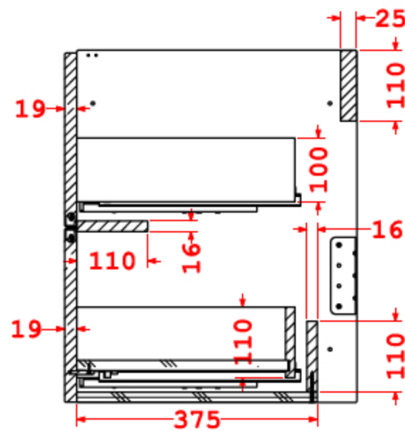
SEZIONE A-A
