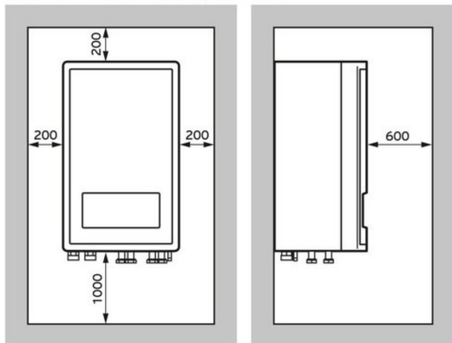
Mindestabstände und Montagefreiräume
