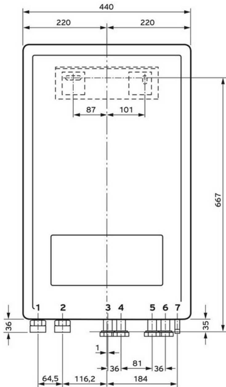
Mindestabstände und Montagefreiräume
