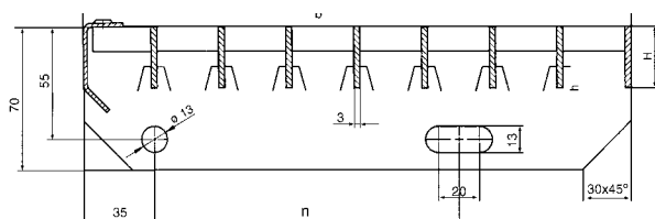
Vue latérale: Marches d'escalier en acier Dimensions de perçage selon DIN 24531
