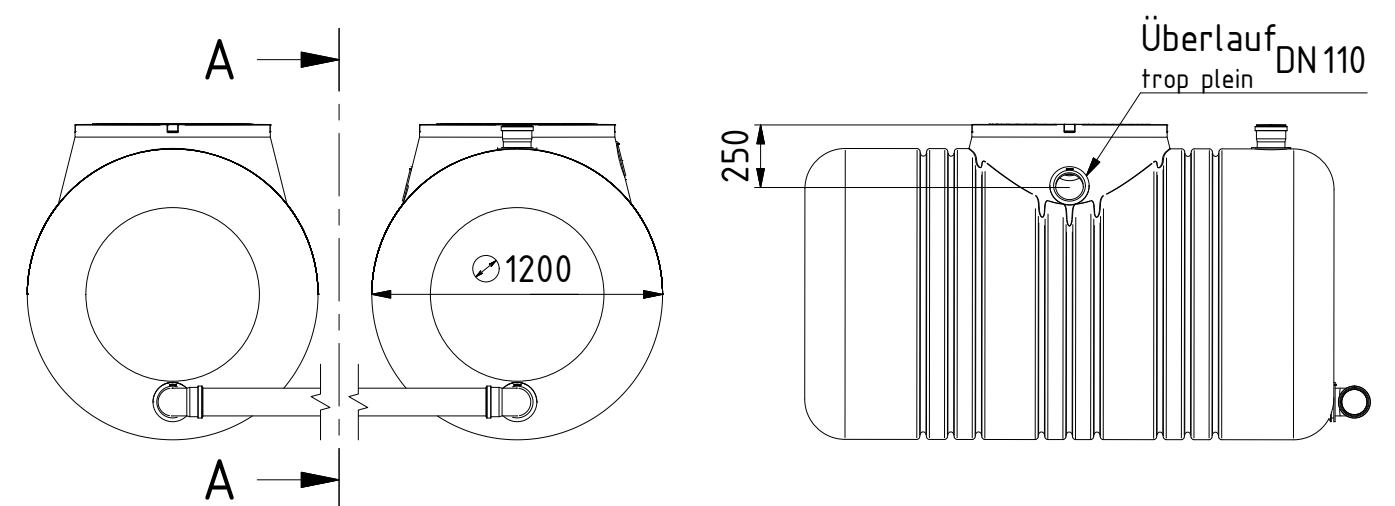
A-A ( 1 : 30 )
