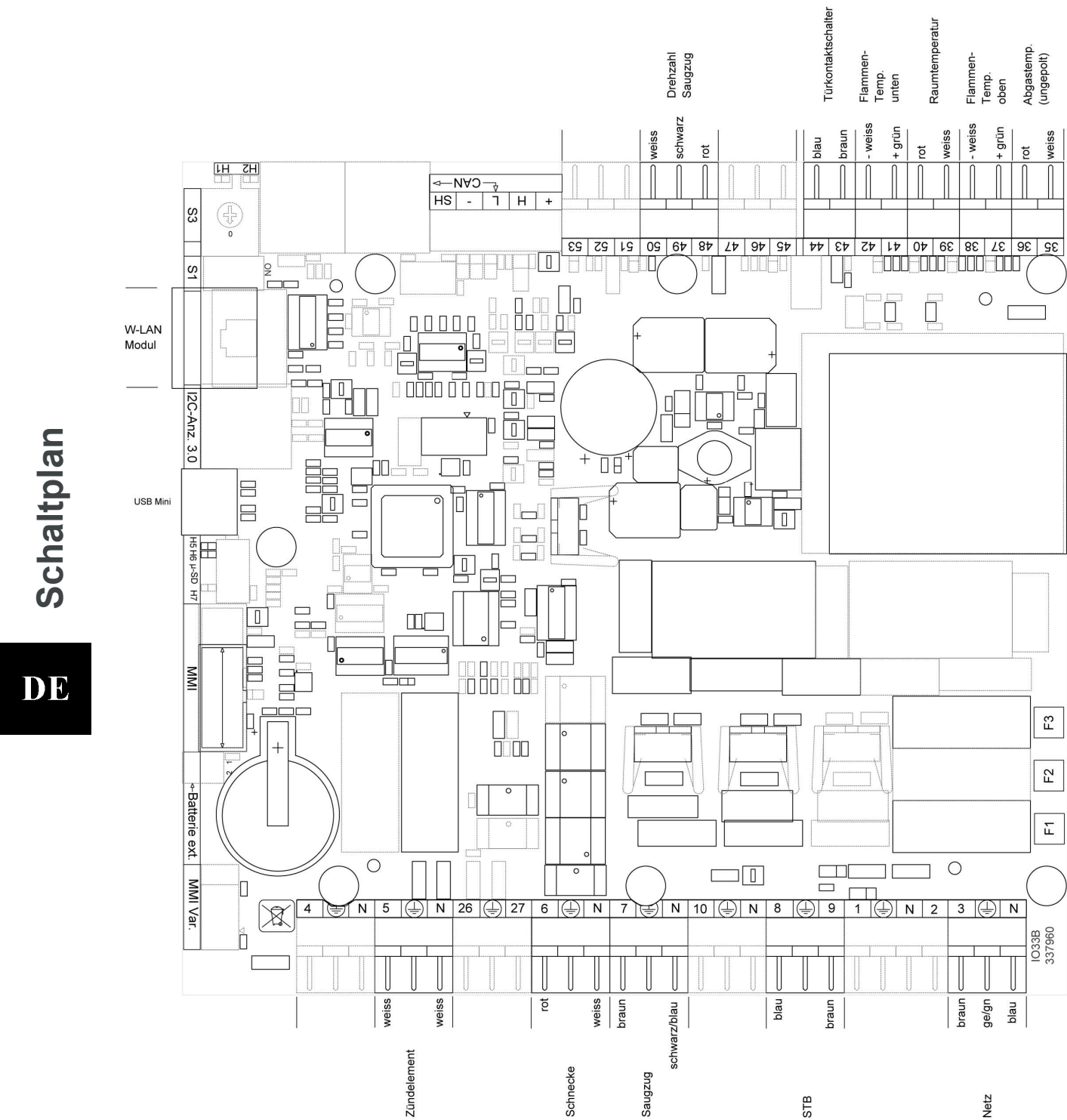
Anschlussplan IO 33.3
