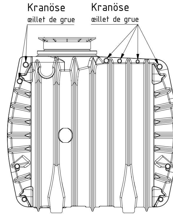
Ansicht von links vue de gauche
