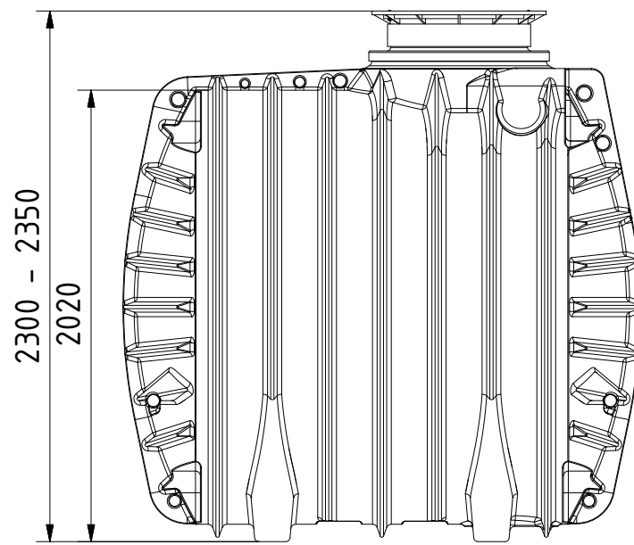
Ansicht von rechts vue de droit
