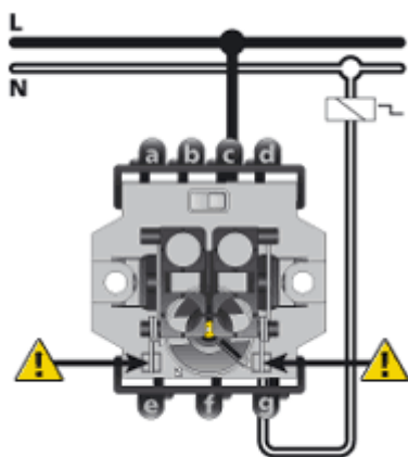
Taster Öffner
