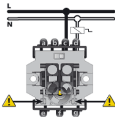
Taster Schließer
