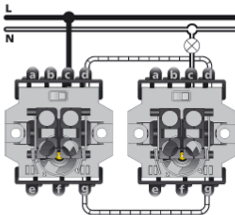
Wechselschaltung
