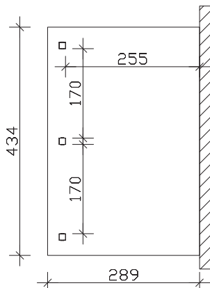
Grundriss
