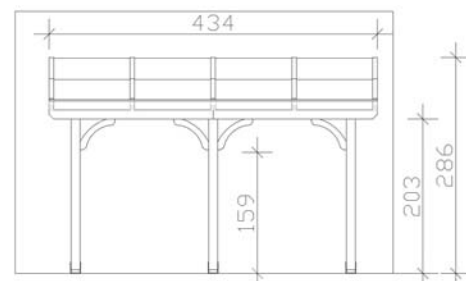
Frontansicht
