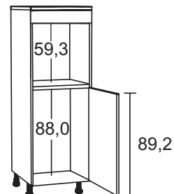
Midischränk für Kühlschrank und Backofen, 1 feste Blende, 1 Drehtür
