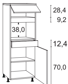
Midischränk für Mikrowelle, 1 Klappe, 1 Schubkasten, 1 Drehtür
