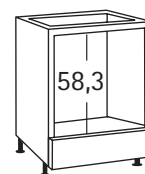
Herdumbau, 1 festen Blende
