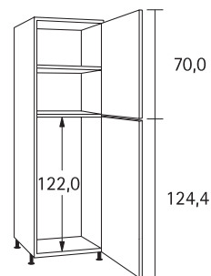
Hochschrank für Kühlschrank, 2 Drehtüren
