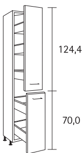
Apothekersschrank, 2 Auszüge mit oben 3 und unten 2 Schubkästen
