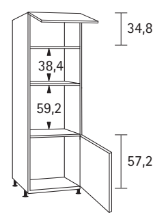
Hochschrank für Mikrowelle und Backofen, 1 Klappe, 1 Drehtür
