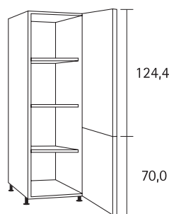
Hochschrank, 2 Drehtüren
