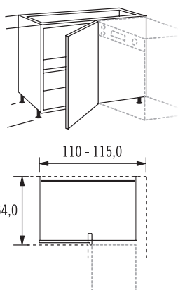
Eckunterschränk, 1 Drehtür
