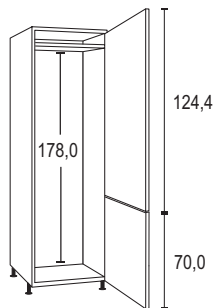
Hochschrank für Kühl-/Gefrierschrank, 2 Drehtüren
