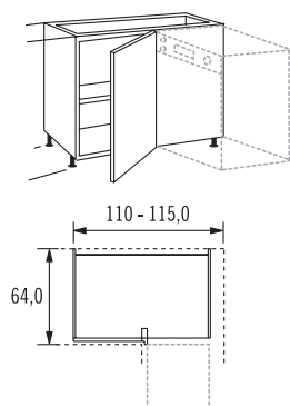
Eckunterschränk, 1 Drehtür
