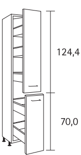
Apothekerschrank, 2 Auszüge mit oben 3 und unten 2 Schubkästen
