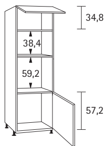
Hochschrank für Mikrowelle und Backofen, 1 Klappe, 1 Drehtür
