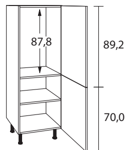
Midischränk für Kühlschrank, 2 Drehtüren
