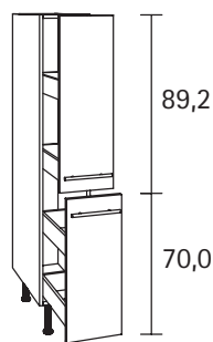
Midi-Apothekerschrank, 2 Auszüge mit je 2 Schubkästen
