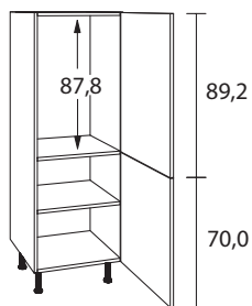
Midischränk für Kühlschrank, 2 Drehtüren
