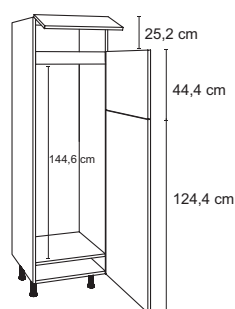
Hochschrank für Kühl-/Gefrierkombination, 1 Klappe, 2 Drehtüren
