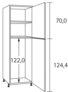
Hochschrank für Kühlschrank, 2 Drehtüren
