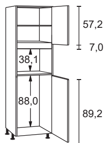
Hochschrank für Mikrowelle und Kühlschrank, 2 Drehtüren
