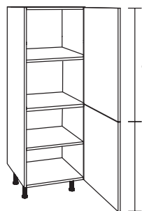
Midischränk, 2 Drehtüren
