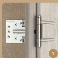
1 Bande de sécurité avec fixation de bande d'acier préparée pour un ancrage mural.
