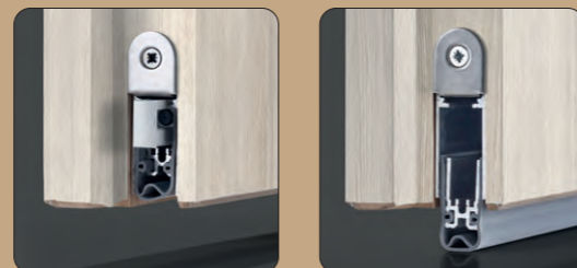
Bodendichtung eingeklappt Bandseite und abgesenkt Schlossseite Jedes Schallschutzelement besitzt eine absenkbare Bodendichtung im Türblatt. Beim Schliessen der Tür wird die Dichtung automatisch abgesenkt.
