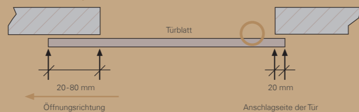
Auf der Anschlagseite beträgt der Überstand durch die Griffmuschel immer 20 mm. Der restliche Überstand bleibt auf der Gegenseite.
