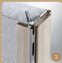
Montagematerial zur Mauerverankerung bauseits zu stellen. (Montagebeispiel für Mauerverankerung).
