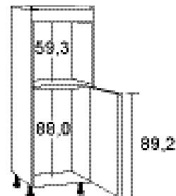
Armoire midi pour réfrigérateur et four, 1 cache fixe, 1 porte pivotante
