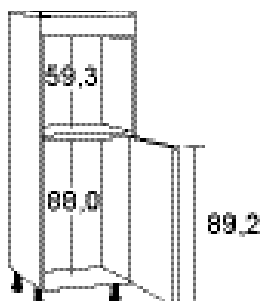
Armoire midi pour réfrigérateur et four, 1 cache fixe, 1 porte pivotante
