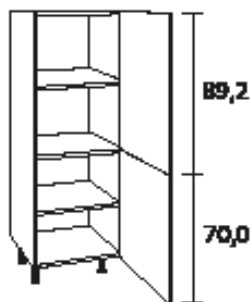
Armoire midi, 2 portes pivotantes
