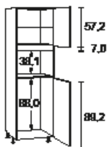
Meuble colonne pour four à micro-ondes et réfrigérateur, 2 portes pivotantes
