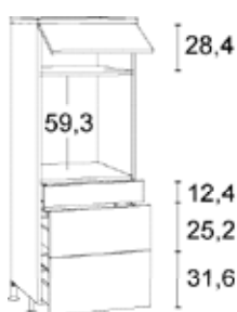
Armoire midi pour four, 1 porte relevable, 1 tiroir, 2 éléments coulissants
