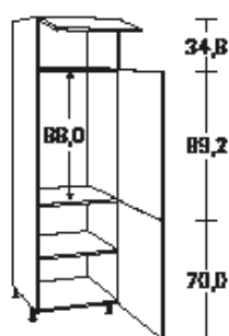
Meuble colonne pour réfrigérateur, 1 porte relevable, 2 portes pivotantes
