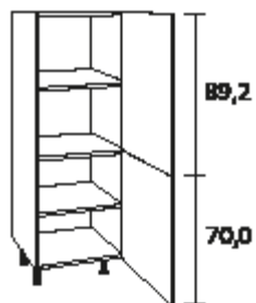
Armoire midi, 2 portes pivotantes
