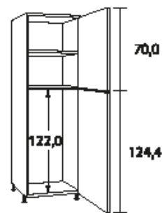
Meuble colonne pour réfrigérateur, 2 portes pivotantes
