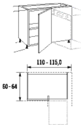
Meuble bas d'angle, 1 porte pivotante
