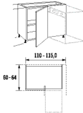
Meuble bas d'angle, 1 porte pivotante
