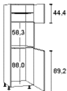
Meuble colonne pour four et réfrigérateur, 2 portes pivotantes
