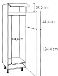
Meuble colonne pour réfrigérateur/congélateur, 1 porte relevable, 2 portes pivotantes
