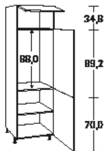
Meuble colonne pour réfrigérateur, 1 porte relevable, 2 portes pivotantes
