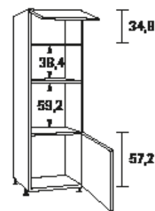
Meuble colonne pour four à micro-ondes et four, 1 porte relevable, 1 porte pivotante
