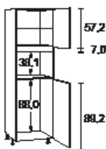
Meuble colonne pour four à micro-ondes et réfrigérateur, 2 portes pivotantes
